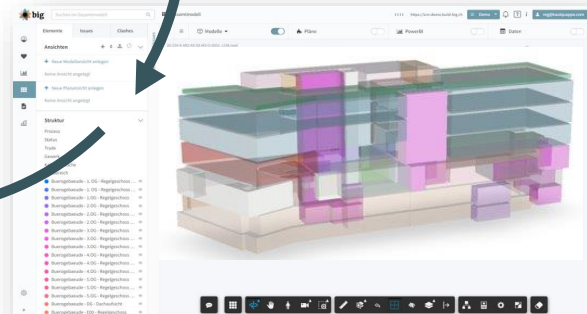
TAKT-Flächenmodell (BIM)
